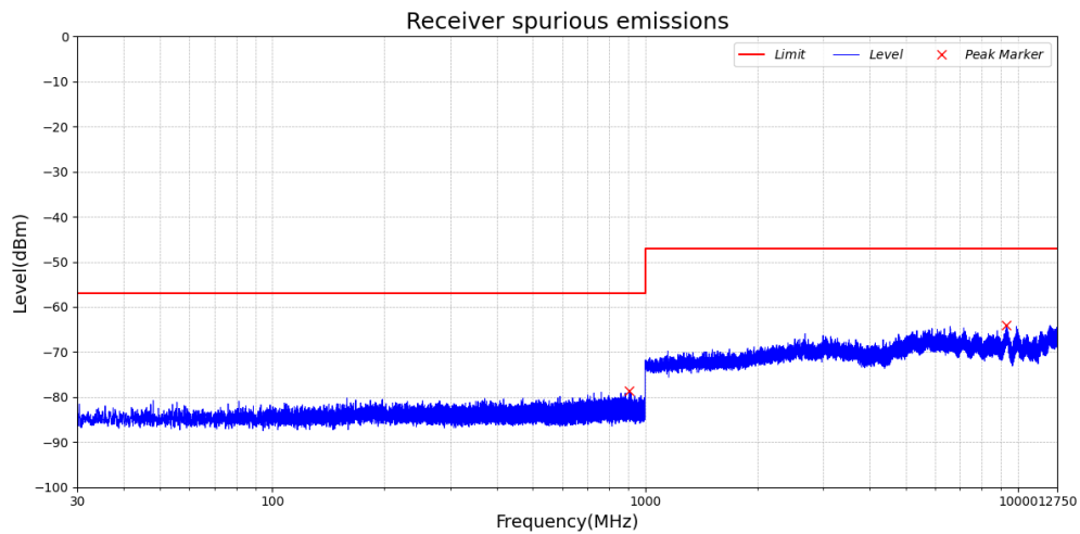
Test_Graph_RX_ANT1_2402_1Mbps
