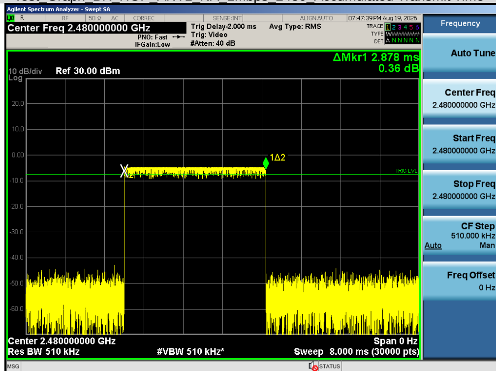
Test_Graph_BR_HOP_ANT1_NA_1Mbps_2480_Burst Time
